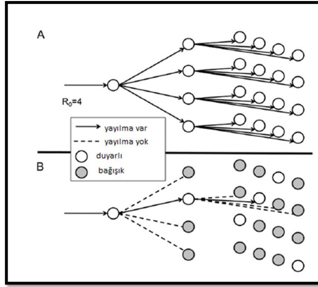
Şekil-12: R_0 4 olan bir enfeksiyonun yayılımını gösteren diyagram
