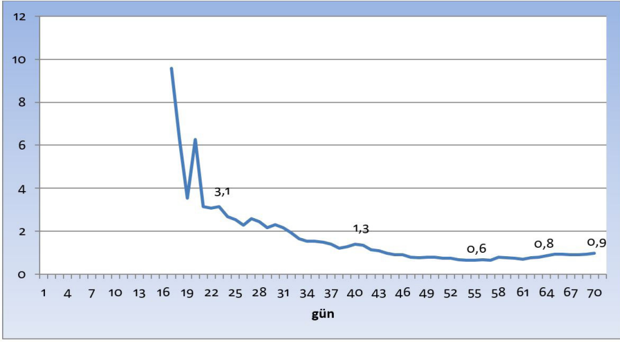
Grafik-17: Türkiye için salgının 18. gününden sonraki tahmini R_0 değerleri ( R_0=erTc ) Tc=7,5 kabul edilmiştir.
