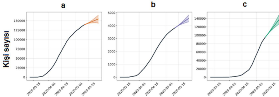
Şekil-B: 15 Günlük zaman serisi tahmini a) toplam vaka sayısı, b) toplam ölüm, c) toplam iyileşme
